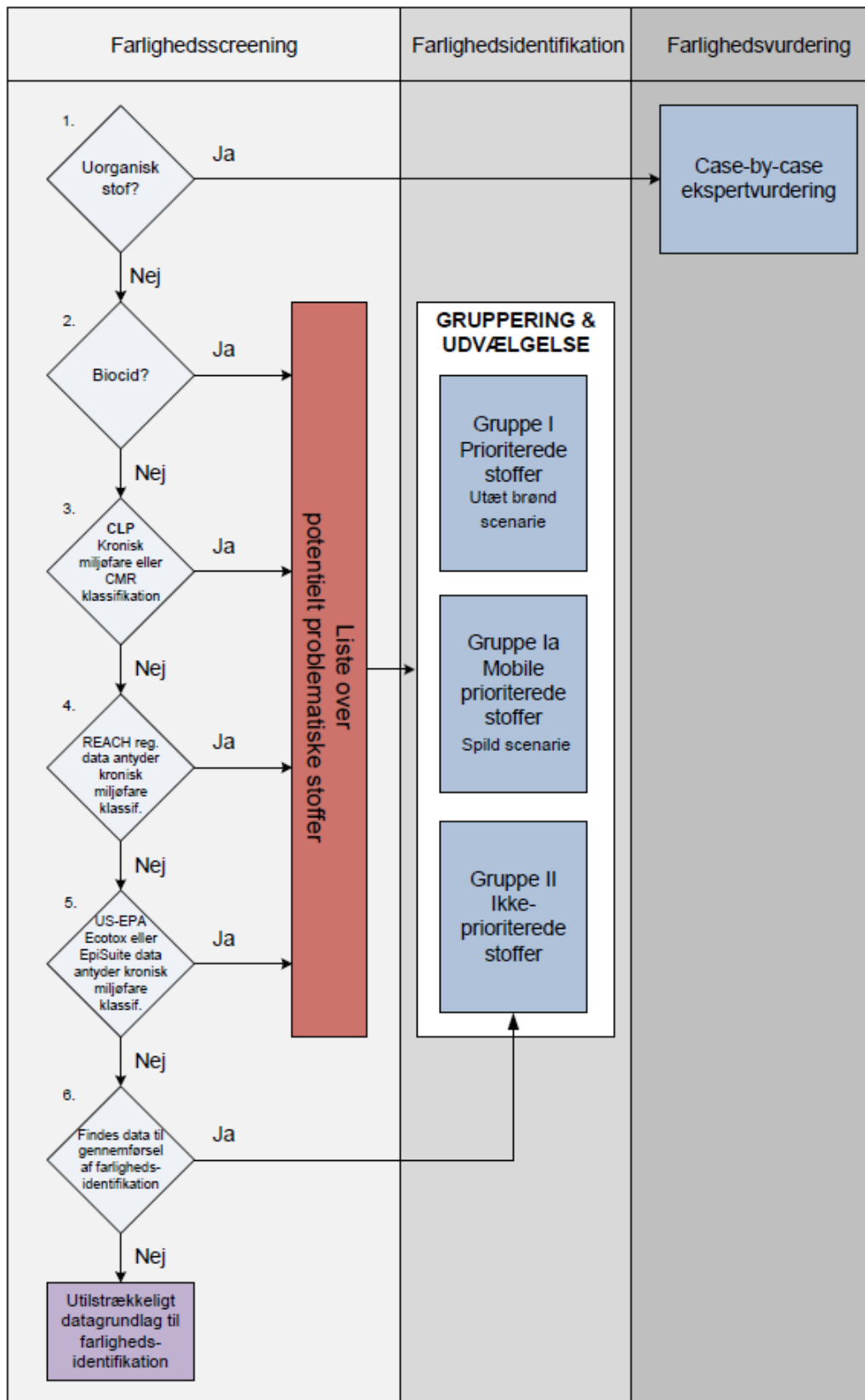
Figur B3. Flowdiagram over sorteringen af kemikalier i boremudder og fraktureringssvæske.
