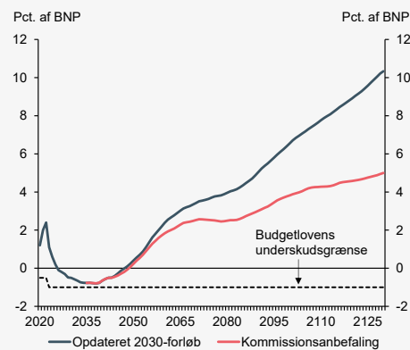
Figur 2 Strukturel saldo
