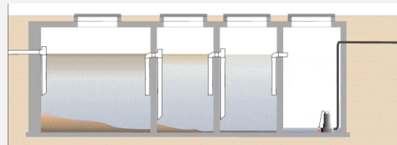
Kilde seperationstank: Samarbejdspartner Janis&Schultz, Tyskland.
