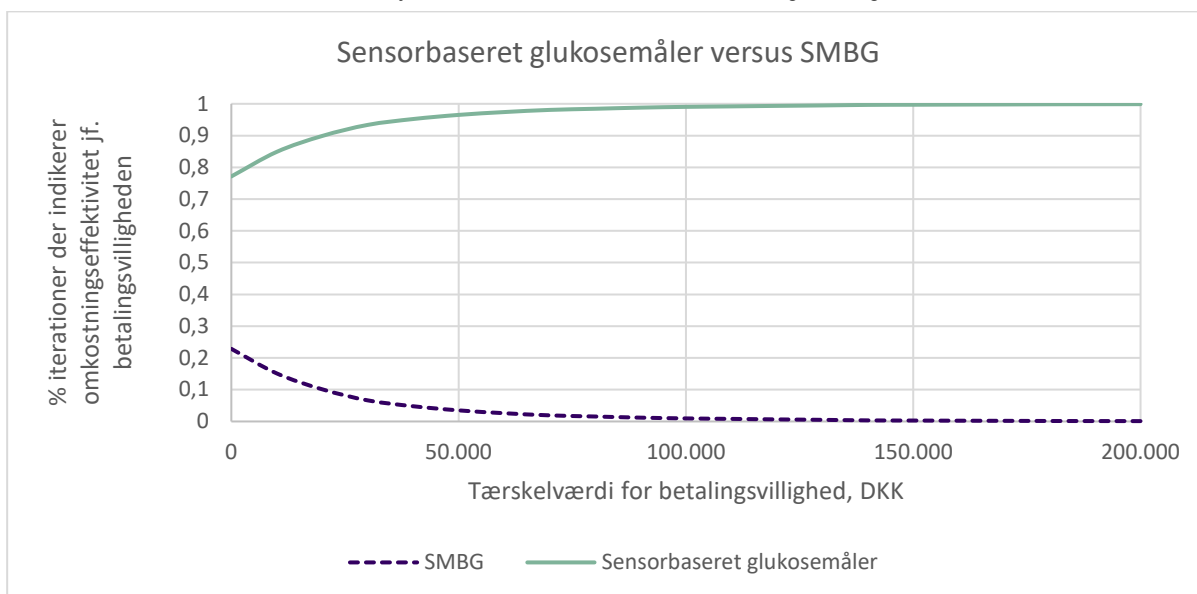
Figur 12 - Cost-effectiveness acceptability kurve. Kurven indikerer sandsynligheden for, at anvendelse af sensorbaseret glukosemåler er omkostningseffektiv set i forhold til anvendelsen af SMBG ved forskellige willingness-to-pay tærskelværdier i cost-utility analysen.
