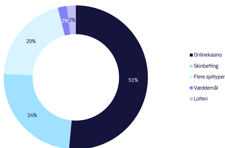
Figur 2. Blokeringer fordelt på spiltyper, 1. halvår 2023
