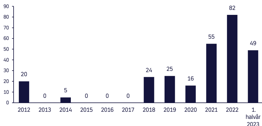
Figur 1. Antal blokerede hjemmesider, 2012- 1. halvår 2023
