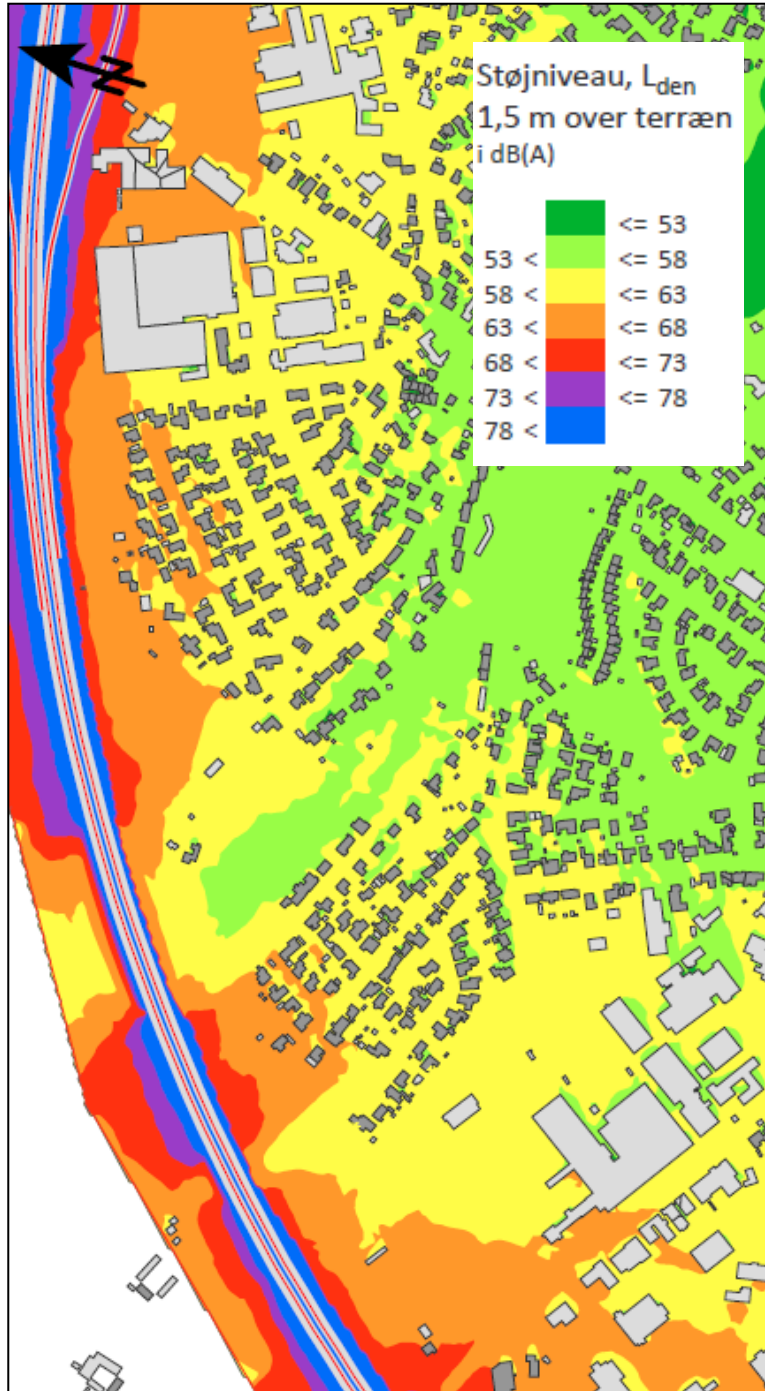
Figur 1 Eksempel på støjkonturkort
