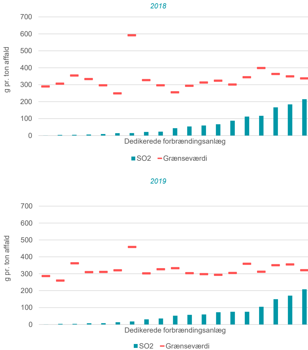
Figur 21a: Udledning af SO 2 , der måles kontinuerligt i g pr. ton affald, 2018 og 2019 (dedikerede forbrændingsanlæg)
