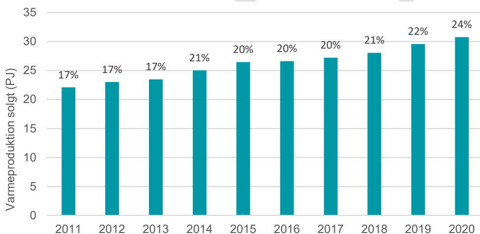
Figur 14a: Forbrændingsanlæggene afsatte produktion af varme, 2011-2020 (pct.-tallet angiver, hvor stor en andel forbrændingsanlæggene produktion udgør af Danmarks samlede fjernvarmeforsyning)
