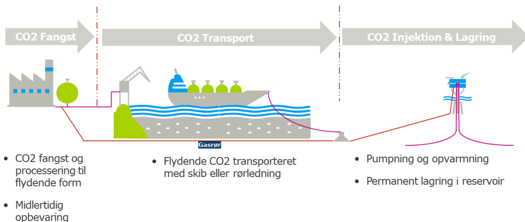
Figur 3-4 Proces fra opsamling til lagring af CO 2 i undergrunden.
