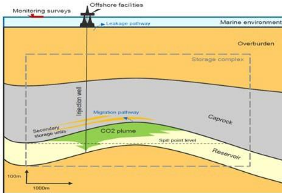
Figur 9-1 CO 2 -lagring i reservoir.
