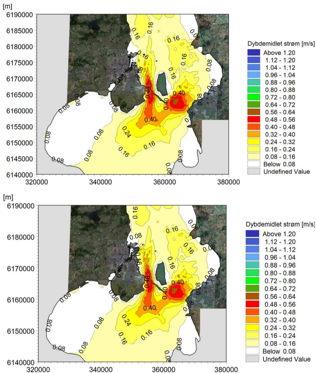
Figur 9 Årsmiddel af dybdemidlet strøm regnet uden retning (bruttostrøm). Øverst: nuværende forhold. Nederst: fremtidige forhold med Lynetteholm.
