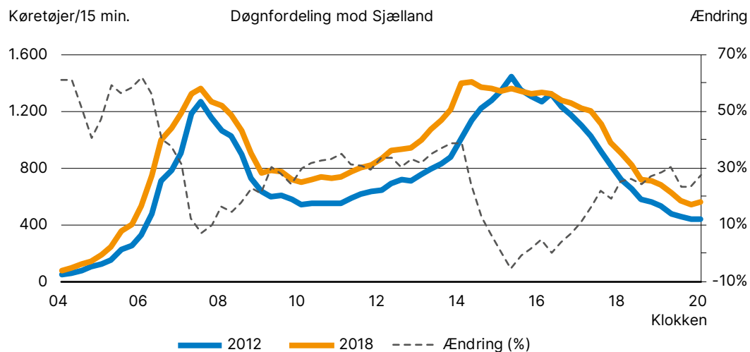
Figur 3.5. Udvikling i døgnfordelingen i retning mod vest ved udfletningen mod henholdsvis Motorring 3 og Køge Bugt Motorvejen. Kilde: Mastra tællinger.
