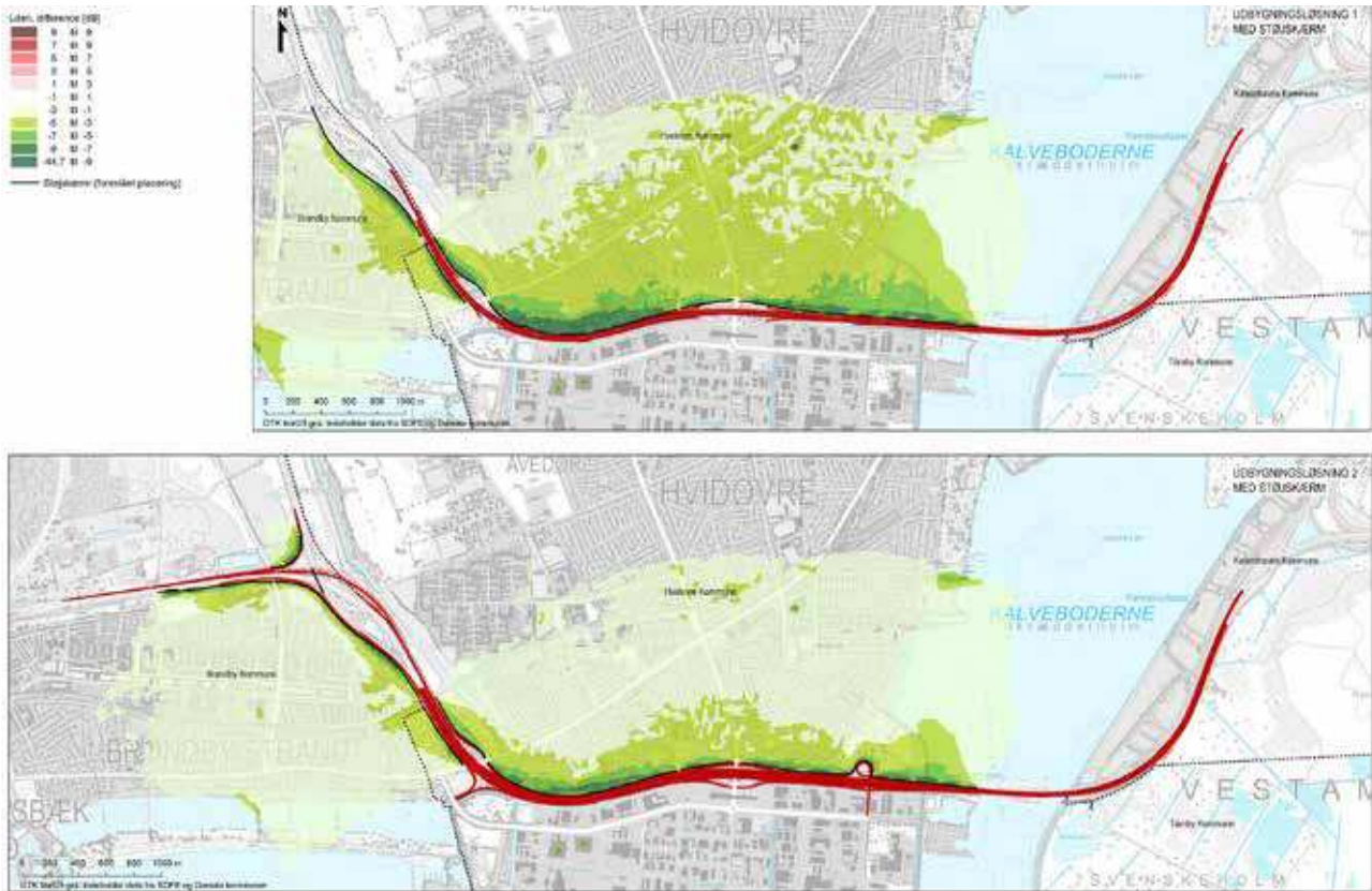
Figur 6.8. Ændringer i støj langs Amagermotorvejen ved udbygningsløsning 1 og 2.
