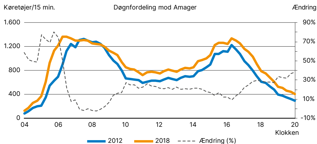
Figur 3.4. Udvikling i døgnfordelingen i retning mod øst ved sammenfletning af Motorring 3 og Køge Bugt Motorvejen. Kilde: Mastra tællinger.
