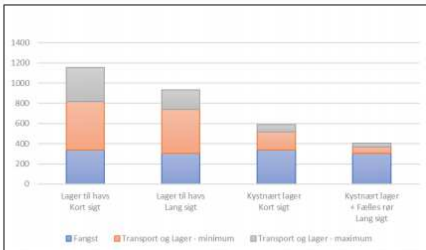
Figur: CO2 omkostninger på kort (før 2030) og på lang sigt (efter 2030) til: (1) fangst, (2) transport + lager til havs eller et kystnaert lager. Lys grå udtrykker forskellige transport og lager modeller samt usikkerhed i prissætning.
