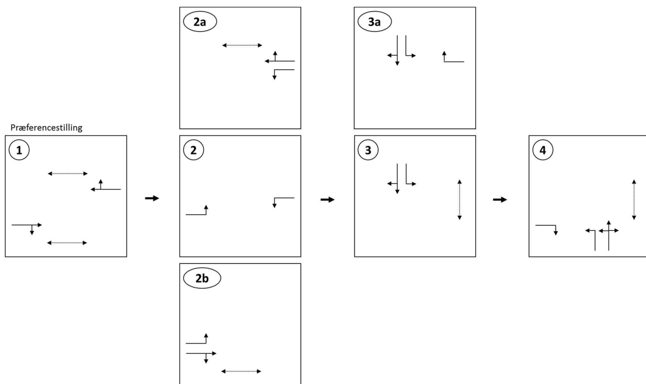
Figur 4.3 Styrediagram for signalafviklingen
