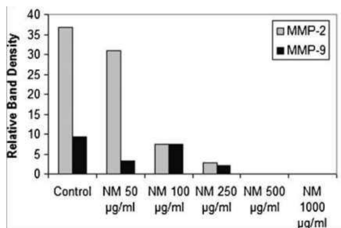
Fig. 5. Måling af MMP-2 og MMP-9 udskillelse fra humane prostata kræftceller. Søjlerne viser, at den udskillelse af MMP-2 og MMP-9, der finder sted ved 0 NM ( Control ) reduceres til 0 ved 500 mikrogram NM pr. milliliter .
