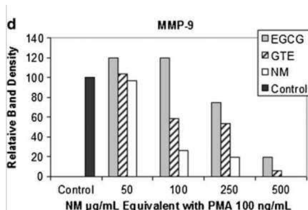
Fig. 2. MMP-9 udskillelse fra humane bindevævsdannende kræftceller.
