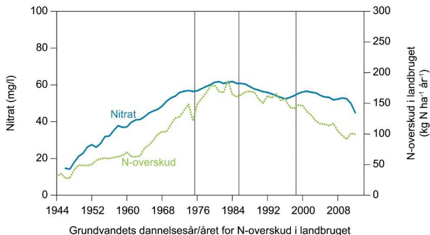
Figur 5.5. Gennemsnitligt nitratindhold som 5-års glidende gennemsnit af i iltet grundvand i forhold til året for grundvandet dannelses og overskud af kvælstof fra landbrugsproduktionen, dvs. den faktuelle nationale kvælstofbalance beregnet for hvert år (Hansen et al. 2017).
