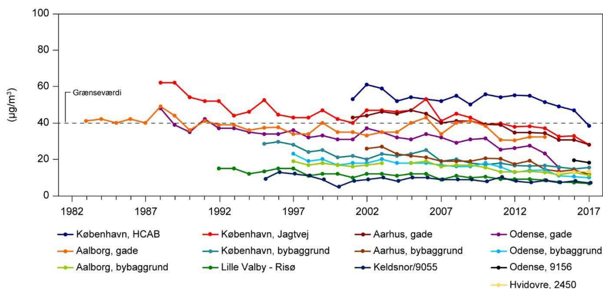
Figur 4.1. Graferne viser tidsserier for årlige gennemsnitsværdier af \text{NO}_2 for de forskellige målestationer. Grænseværdien er 40 \mu\text{g}/\text{m}^3 og trådte i kraft i 2010 (Ellermann et al. 2018).
