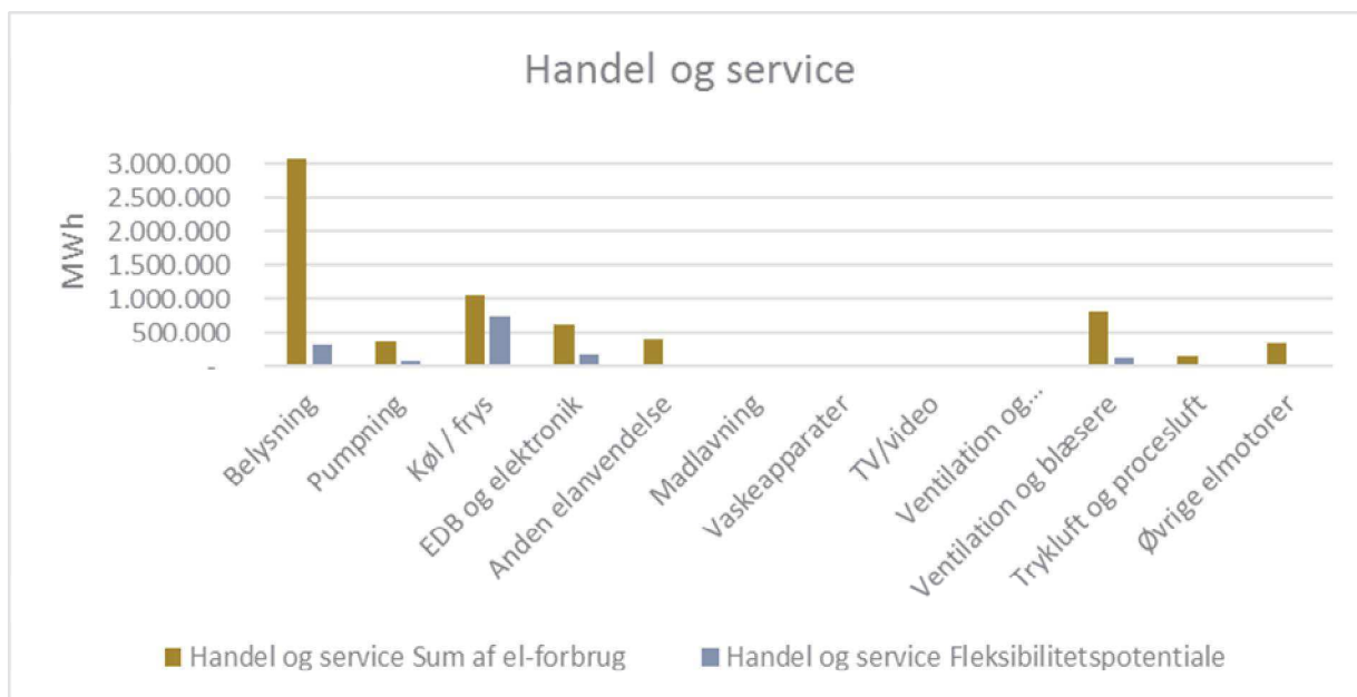
Figur 10: Opgjort fleksibilitetspotentiale for el (ekskl. el til opvarmning) for handel og service opdelt på anvendelse.
