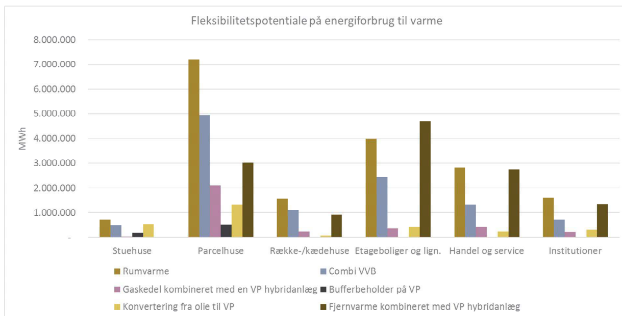
Figur 2: Opgjort fleksibilitetspotentiale på varmesiden opdelt på bygningstype og tiltag.
