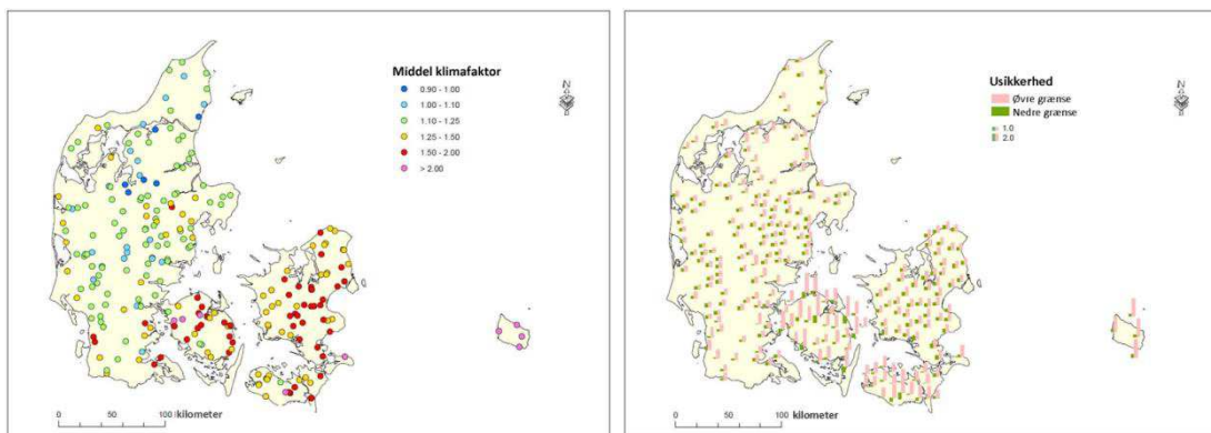
Figur 5.8. Figuren viser klimafaktorer for klimabetinget ændring i 100-års maksimumafstrømning vurderet for perioden 2021-2050 i forhold til perioden 1961-1990 (til venstre) og beregnede usikkerhedsbånd (til højre). Klimafaktoren angiver, hvor meget større/mindre maksimumafstrømningen bliver i det fremtidige klima sammenlignet med 1961-1990. Kilde: GEUS 5 .
