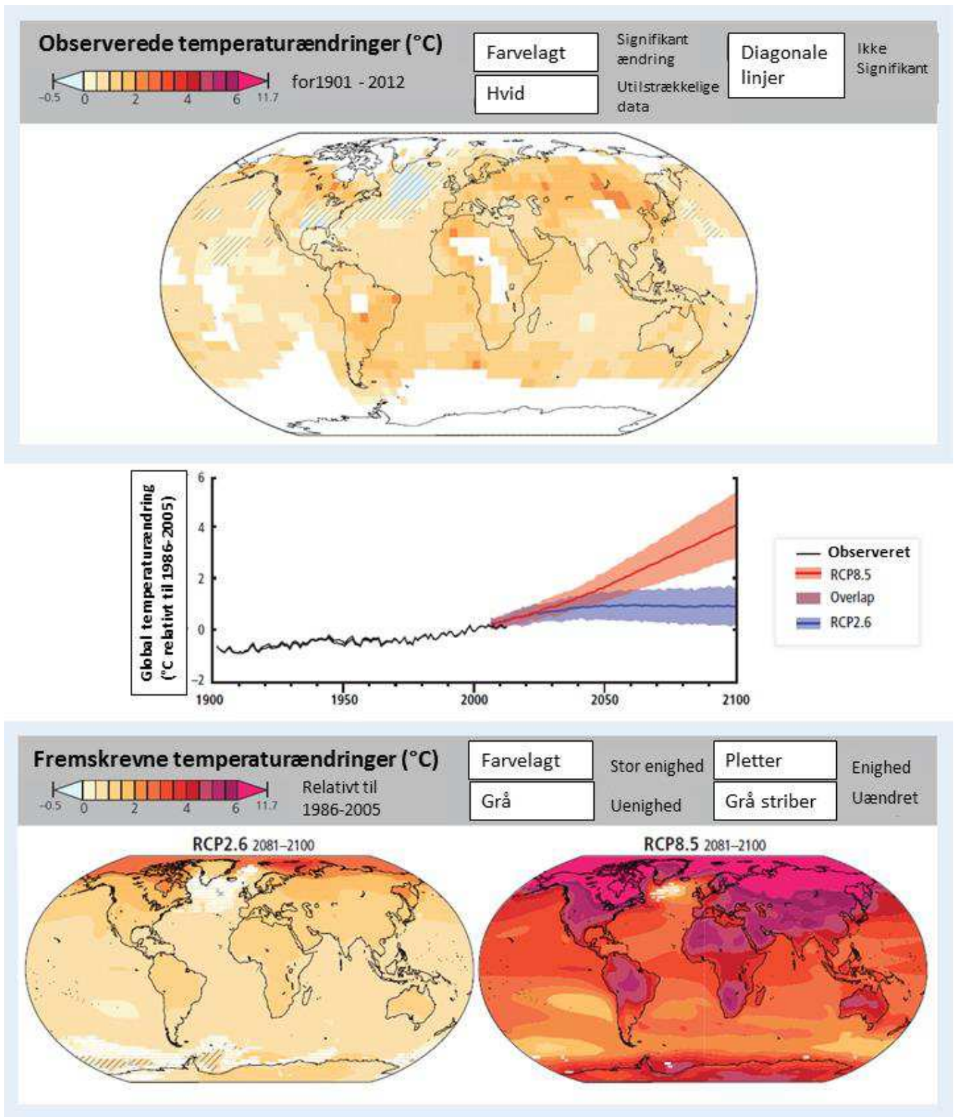
Figur 5.1. Figuren viser (øverst) et kort over årlige temperaturændringer fra 1901-2012. Hvide områder viser, at datagrundlaget ikke er tilstrækkeligt. Områder, hvor tendensen ikke er signifikant, er skraverede. Figuren i midten viser observerede og simulerede fremtidige temperatur i forhold til perioden 1986-2005. Nederste kort viser temperaturændringer i RCP2.6 og RCP8.5 set i forhold til 1986-2005. Kilde: IPCC
