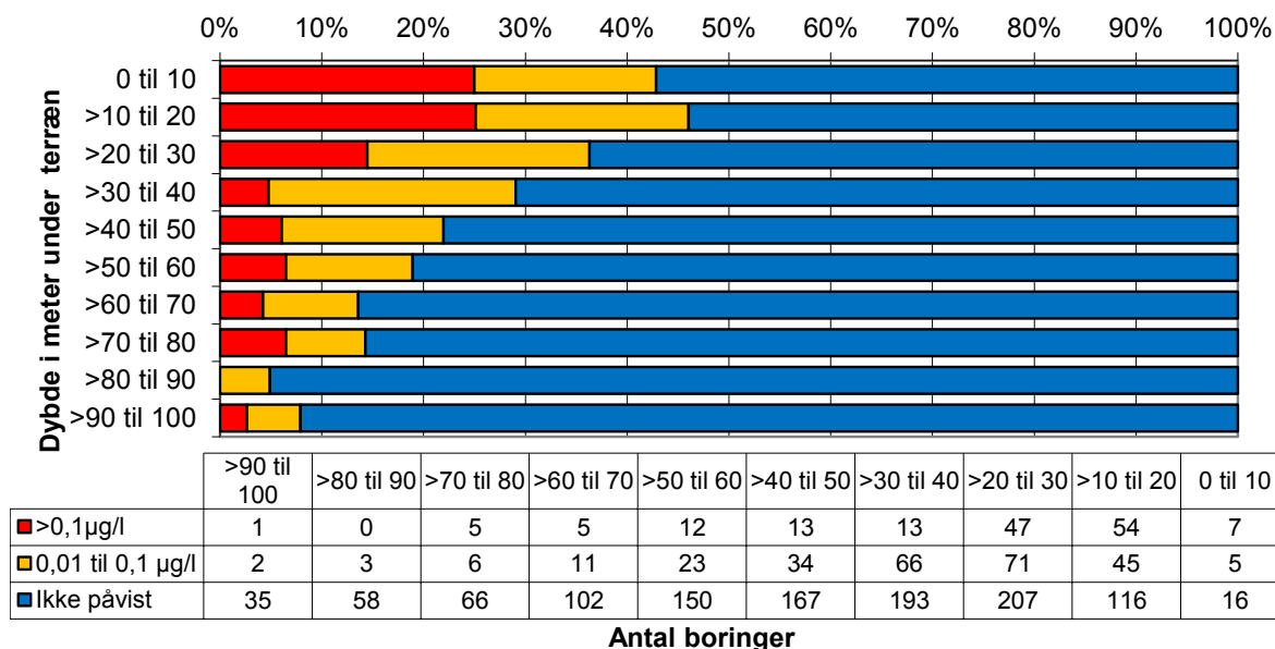
Figur 4. Boringskontrollen. Desphenylchloridazons dybdefordeling. Boringerne er opdelt i tre koncentrationsintervaller: mindst én overskridelse af grænseværdien for drikkevand (>0,1 µg/l), mindst ét fund under grænseværdien (0,01-0,1 µg/l), samt ikke påvist (under detektionsgrænsen på <0,01µg/l). Dybden angiver afstanden fra terræn til overkanten af filteret.
