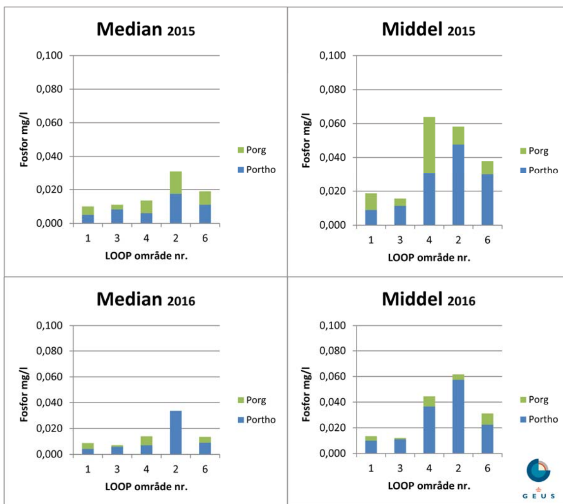
Figur 52. Indholdet af fosfor (mg/l) i det øvre grundvand opdelt på P_{ortho} og P_{org} for de enkelte LOOP-områder i 2015 og 2016. For hvert LOOP område er beregnet hhv. middelværdien og median af hhv. årlige middelværdier og medianer på indtagsniveau.
