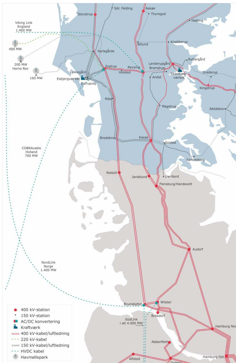
Figur 4: Vestkystforbindelsen fra Endrup via Niebüll til Brunsbüttel.
