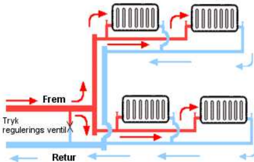
Eksempel på 2-strengsanlæg
