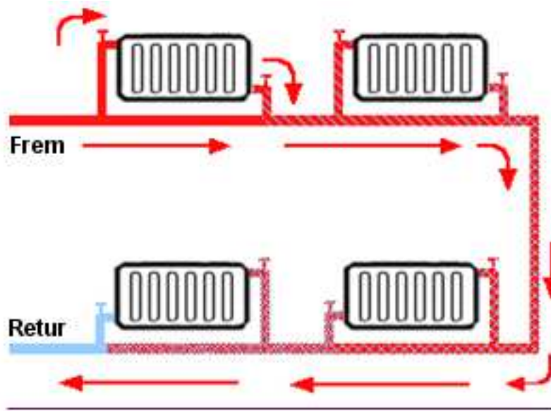
Eksempel på 1-strengsanlæg
