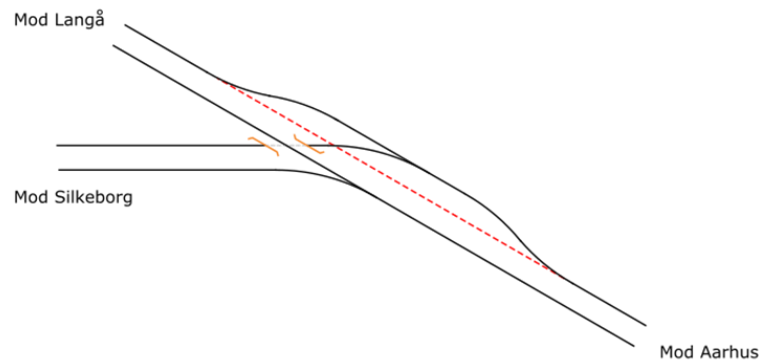
Figur 21. Niveaufri tilslutning til hovedbanen.
