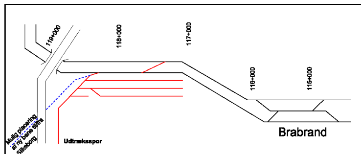
Figur 73. Schematisk sporplan for evt. sportilslutning med enkeltsporet bane til Silkeborg (sorte linjer er hovedbanen Aarhus-Aalborg, blå linjer ny bane til Silkeborg, røde linjer transversal og evt. ny kombiterminal)
