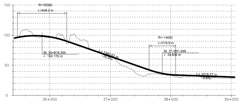
Figur 13. Længeprofil for banen ned mod Svejlbæk. Over en strækning på ca. 2 km er der en højdeforskel på ca. 70 m.
