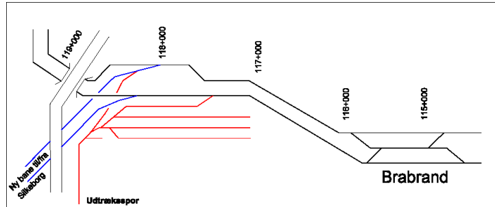
Figur 72. Schematisk sporplan for evt. sportilslutning med dobbeltsporet bane til Silkeborg (sorte linjer er hovedbanen Aarhus-Aalborg, blå linjer ny bane til Silkeborg, røde linjer evt. ny kombiterminal.)
