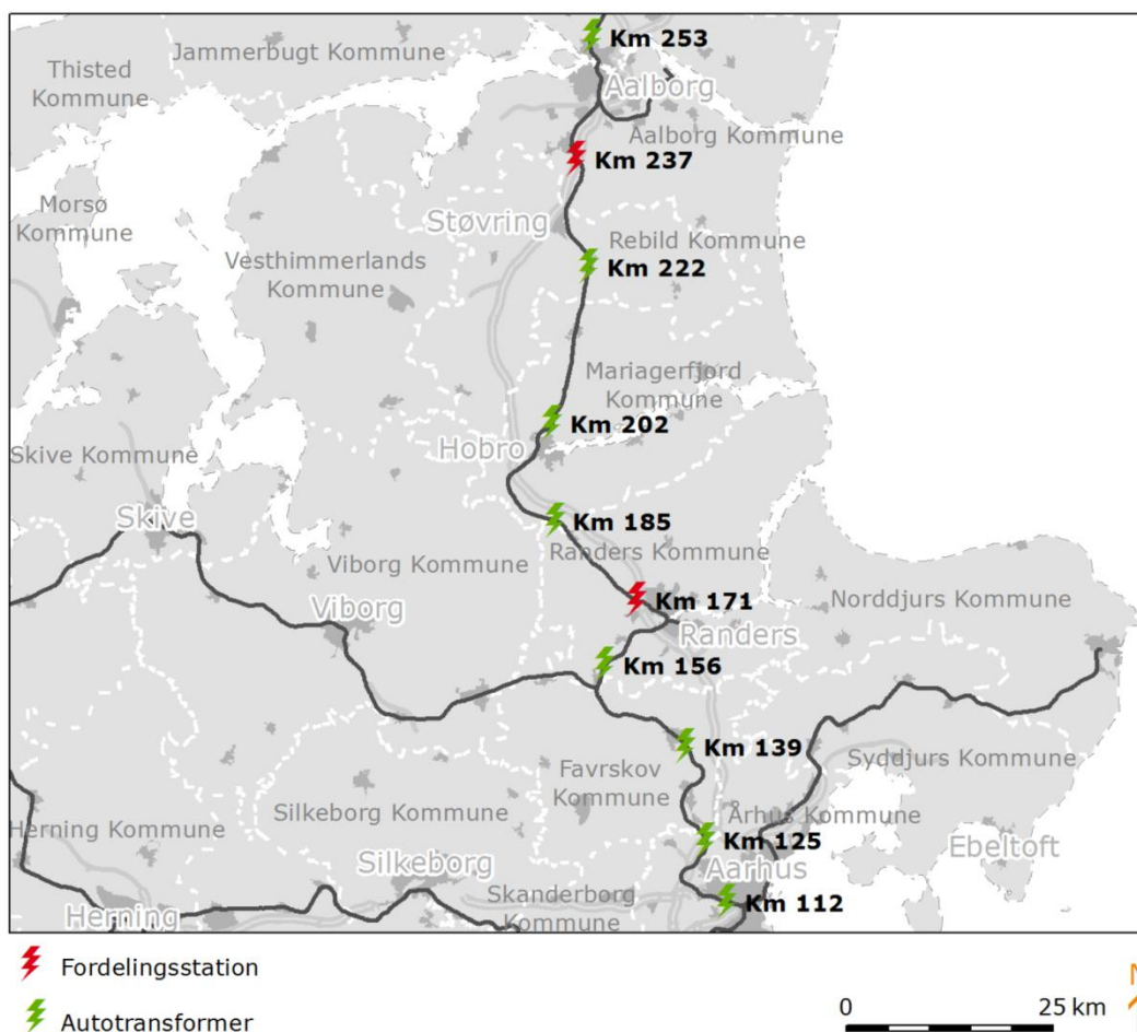
Fig. 3. Fordelingsstationer og autotransformere.
