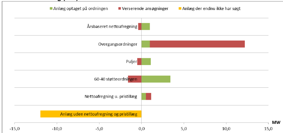
Figur 2: Ændringer i udbygningen på de forskellige ordninger siden sidste månedsstatistik – nettilsluttede anlæg (MW)
