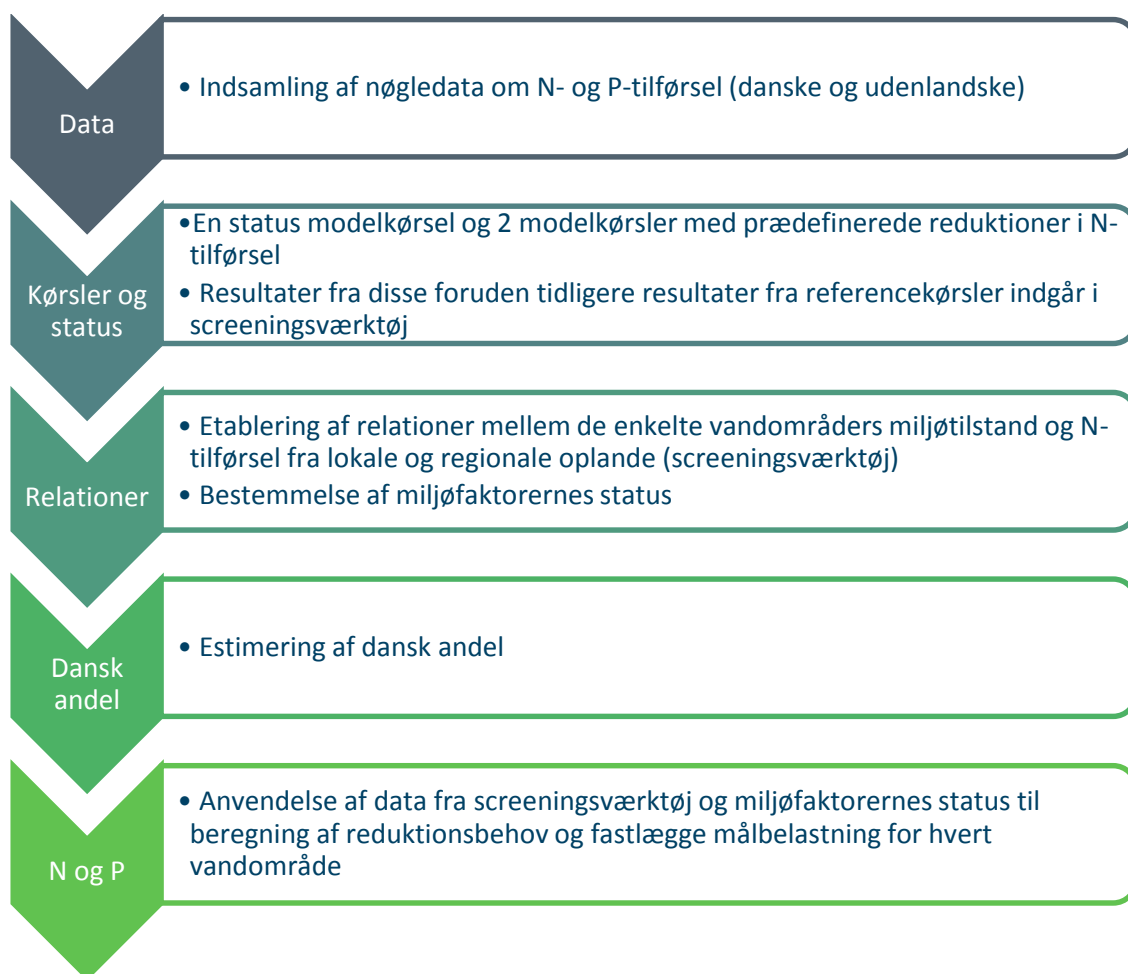
Figur 1 Opsumming af arbejdsgangen for anvendelse af de mekanistiske modeller til vurdering af målbelastninger og reduktionsbehov.
