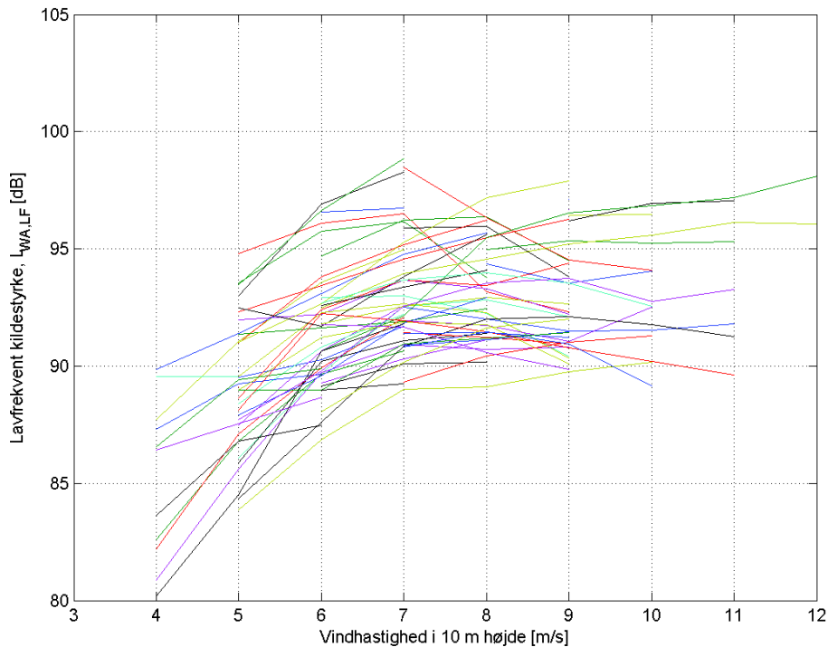
FIGUR 23 DEN LAVFREKVENTE KILDESTYRKE SOM FUNKTION AF VINDHASTIGHEDEN FOR ALLE VINDMØLLER DER KØRER I STØJREDUCERET INDSTILLING.
