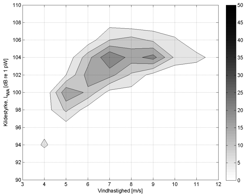
FIGUR 19 KONTOURPLOT PÅ BAGGRUND AF HISTOGRAM FOR VINDMØLLER I STØJREDUCERET INDSTILLING .
