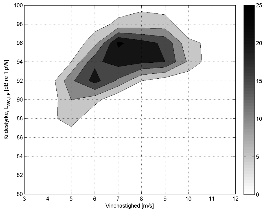
FIGUR 33 KONTOURPLOT PÅ BAGGRUND AF HYPPIGHEDEN AF DE FORSKELLIGE LAVFREKVENTE KILDESTYRKER FOR VINDMØLLER I STANDARDSTØJINDSTILLING.
