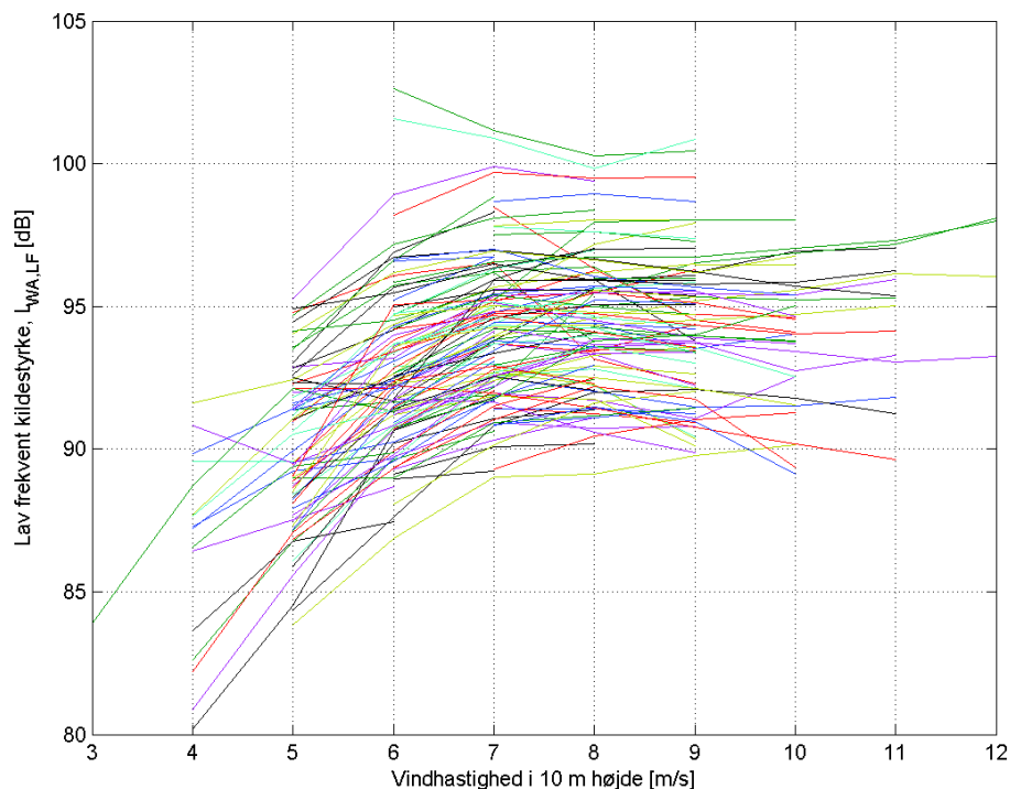
FIGUR 20 SAMLET OVERBLIK OVER ALLE DE FUNDNE DATA I DET LAVFREKVENTE FREKVENSBOMRÅDE. HER VISES DEN LAVFREKVENTE KILDESTYRKE SOM FUNKTION AF VINDHASTIGHEDEN.
