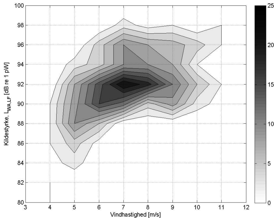
FIGUR 34 KONTOURPLOT PÅ BAGGRUND AF HYPPIGHEDEN AF DE FORSKELLIGE LAVFREKVENTE KILDESTYRKER FOR VINDMØLLER I STØJREDUCERET INDSTILLING.
