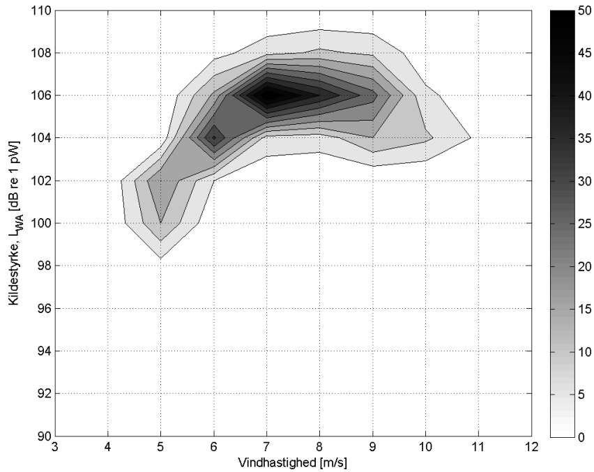
FIGUR 18 KONTOURPLOT PÅ BAGGRUND AF HISTOGRAM FOR VINDMØLLER I STANDARDSTØJINDSTILLING .
