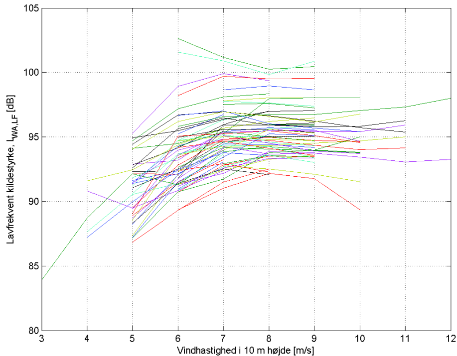
FIGUR 22 DEN LAVFREKVENTE KILDESTYRKE SOM FUNKTION AF VINDHASTIGHEDEN FOR ALLE VINDMØLLER DER KØRER I STANDARDSTØJINDSTILLING.
