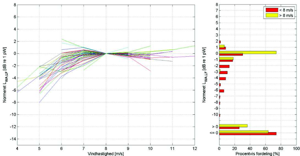
FIGUR 26 DEN NORMEREDE LAVFREKVENTE VINDMØLLESTØJEN SOM FUNKTION AF VINDHASTIGHEDEN RELATIVT TIL KILDESTYRKEN VED 8 M/S FOR VINDMØLLER I STANDARDSTØJINDSTILLING.
