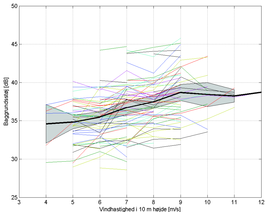
FIGUR 36 UDVIKLINGEN AF BAGGRUNDSSTØJEN SOM FUNKTION AF VINDHASTIGHEDEN FOR SAMTLIGE 74 MÅLINGER SAMT MIDDELVÆRDI OG 95 % KONFIDENSINTERVAL (HHV. FED SORT OG GRÅT AREAL).
