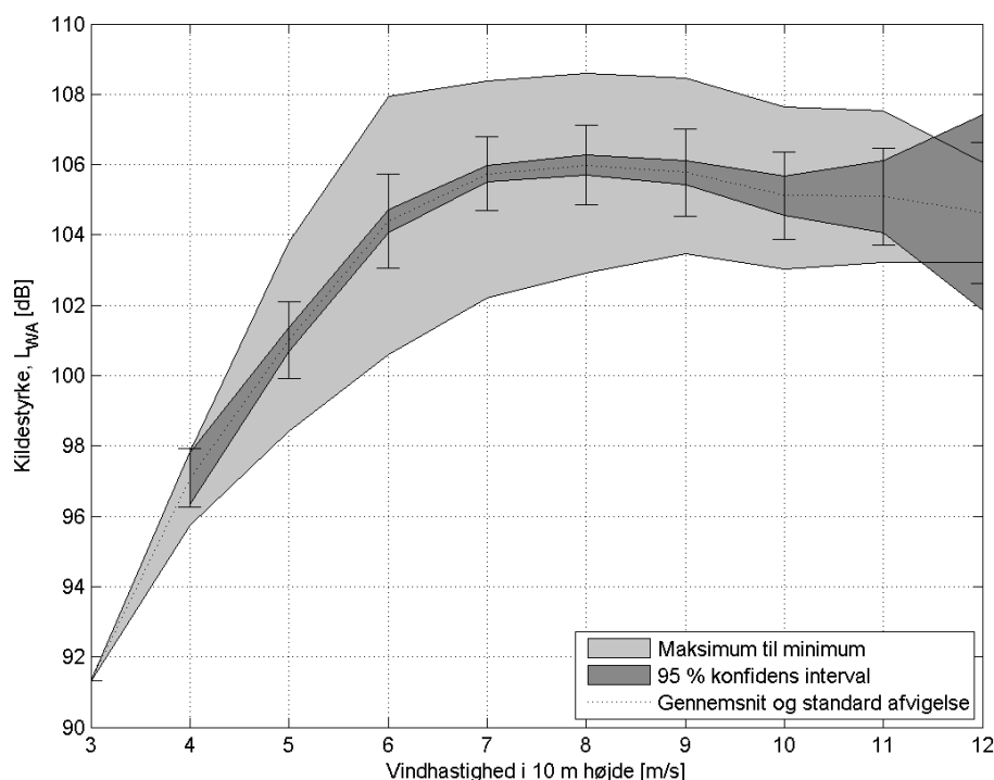
FIGUR 15 VINDMØLLESTØJEN SOM FUNKTION AF VINDHASTIGHEDEN FOR VINDMØLLER I STANDARDSTØJINDSTILLING. FIGUREN VISER MIDDELVÆRDI, STANDARDAFVIGELSE, MAKSIMALVÆRDI, MINIMALVÆRDI SAMT KONFIDENSINTERVAL FOR HVER VINDHASTIGHED.
