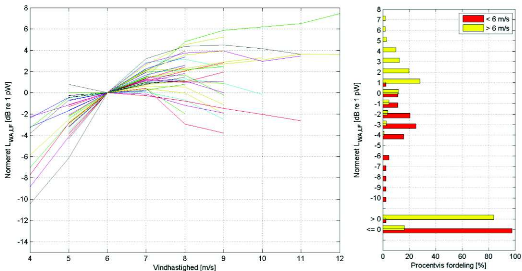
FIGUR 27 DEN NORMEREDE LAVFREKVENTE VINDMØLLESTØJ SOM FUNKTION AF VINDHASTIGHEDEN RELATIVT TIL KILDESTYRKEN VED 6 M/S FOR VINDMØLLER I STØJREDUCERET INDSTILLING.
