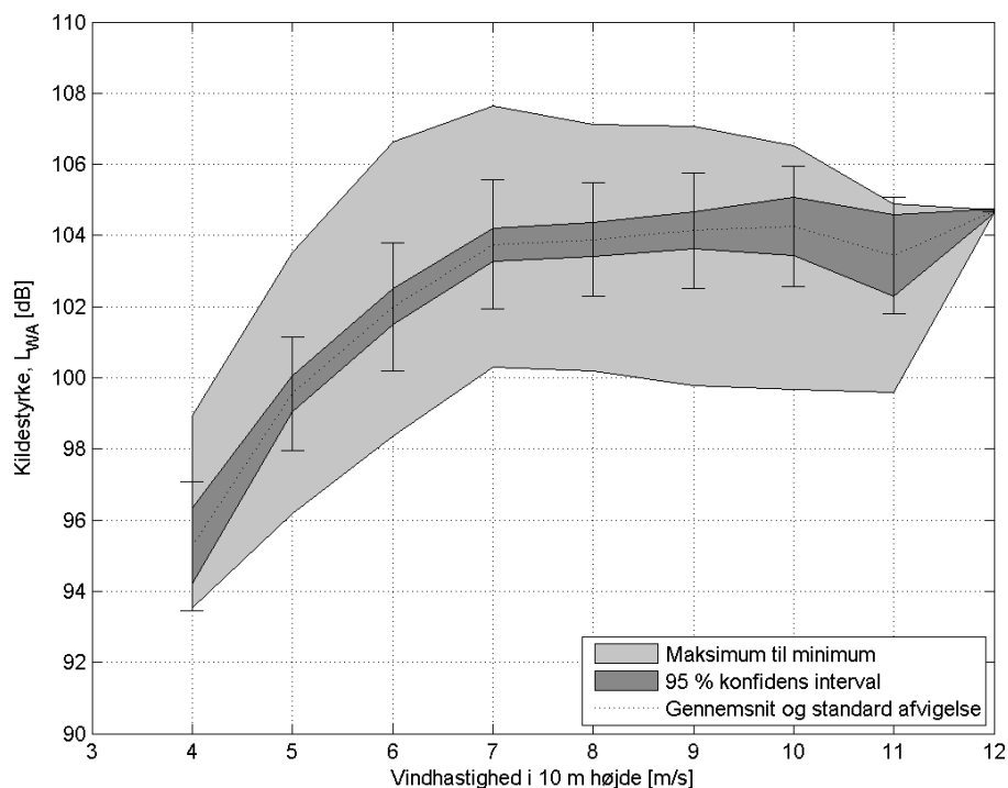
FIGUR 16 VINDMØLLESTØJEN SOM FUNKTION AF VINDHASTIGHEDEN FOR STØJREDUCEREDE VINDMØLLER. FIGUREN VISER MIDDELVÆRDI, STANDARDAFVIGELSE, MAKSIMALVÆRDI, MINIMALVÆRDI SAMT KONFIDENSINTERVAL FOR HVER VINDHASTIGHED
