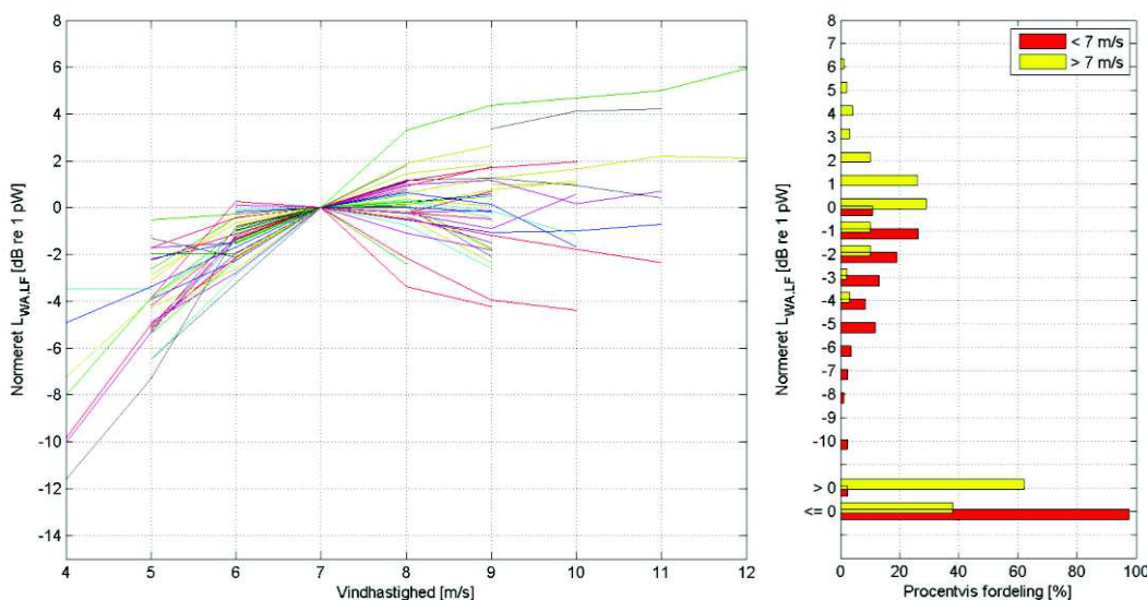
FIGUR 28 DEN NORMEREDE LAVFREKVENTE VINDMØLLESTØJ SOM FUNKTION AF VINDHASTIGHEDEN RELATIVT TIL KILDESTYRKEN VED 7 M/S FOR VINDMØLLER I STØJREDUCERET INDSTILLING.
