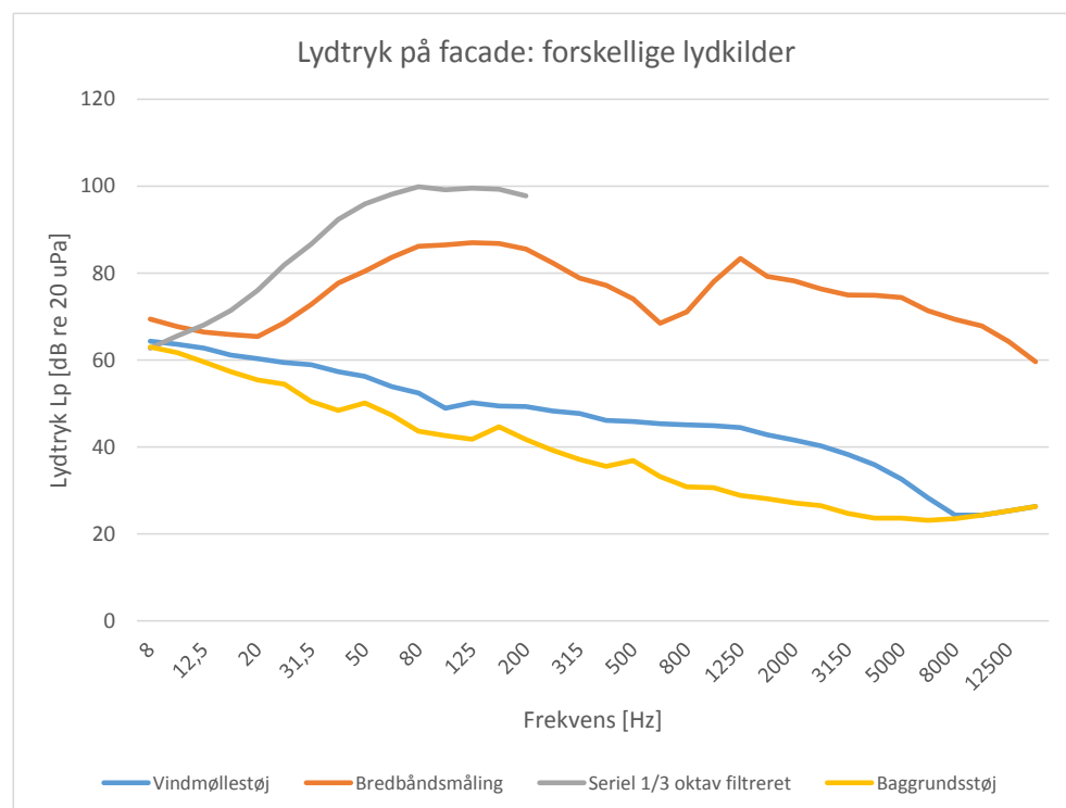
Figur 6. Sammenligning af lydtryk på facade målt med forskellige lydkilder, højtaler på terræn og vindmølle. Til sammenligning er baggrundsstøjen vist. Baggrundsstøjen indgår i kurverne for både vindmøllestøj og højtalerstøj. Kurverne er uden frekvensvægtning (Lineære)
