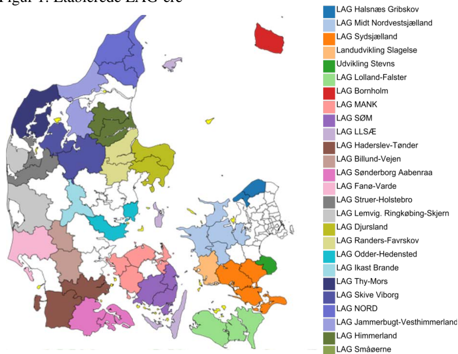
Figur 1: Etablerede LAG'ere
