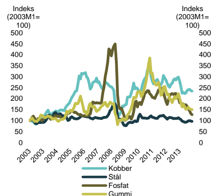
Figur 2. Stål-, kobber-, fosfat- og gummipriser deflateret med løn, 2003-2013
