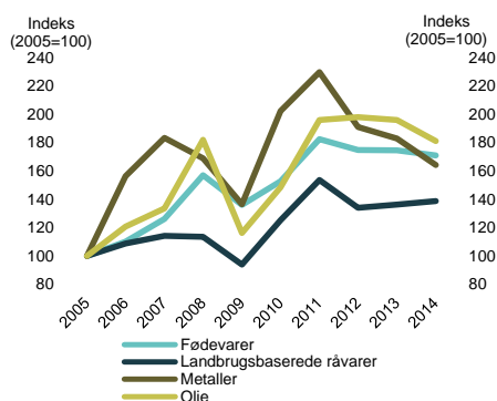
Figur 1. Udviklingen i råvarepriser, 2005-2014
