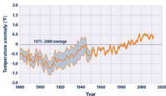
FIGUR 5.4.4 Gennemsnitstemperaturen i verdenshavene, 1880-2012 [7].
