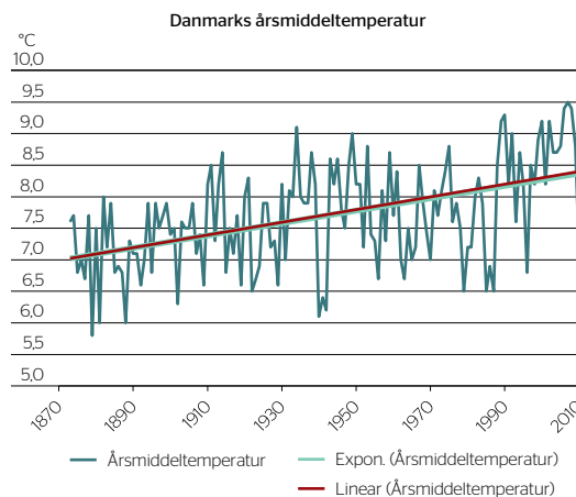
FIGUR 5.3.1 Årsmiddeltemperatur fra 1873-2012. Den røde kurve viser middelværdier [2].
