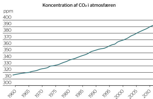
FIGUR 5.2.1 Koncentrationen af CO 2 (kuldioxid) i atmosfæren fra 1959 til 2012 er målt i ppm (parts per million). Målingerne foretages på Hawaii på Mauna Loa Vulkanen i 3,4 km's højde.
