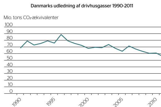
FIGUR 5.1 Danmarks udledning af drivhusgasser fra 1990 til 2011 [4].
