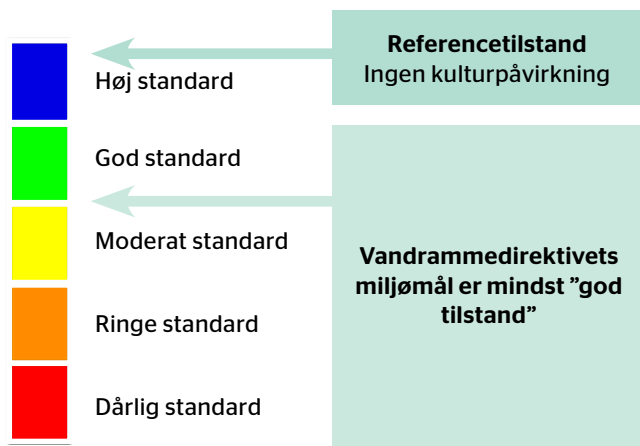
FIGUR 3.11 Vandrammedirektivets målsætningssystem.
