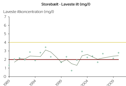
FIGUR 4.2.2 Laveste iltkoncentration i bundvandet i august-oktober i sydlige Kattegat og i det nordlige Storebælt i de sidste 20-30 år. Vandrette orange og røde linjer viser niveauer for iltsvind (< 4 mg ilt/l) og kraftigt iltsvind (< 2 mg ilt/l). Kurverne viser langtidstendensen (3-års glidende gennemsnit) [3].
