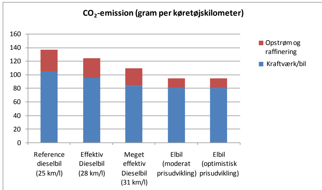
Figur 7: CO 2 -emissioner per køretøjskilometer for hhv. dieselbiler (25 km/l, 28 km/l og 31 km/l) og elbiler i 2020. Tallene ekskluderer opstrømmissioner og tab forbundet med raffinering af diesel.
