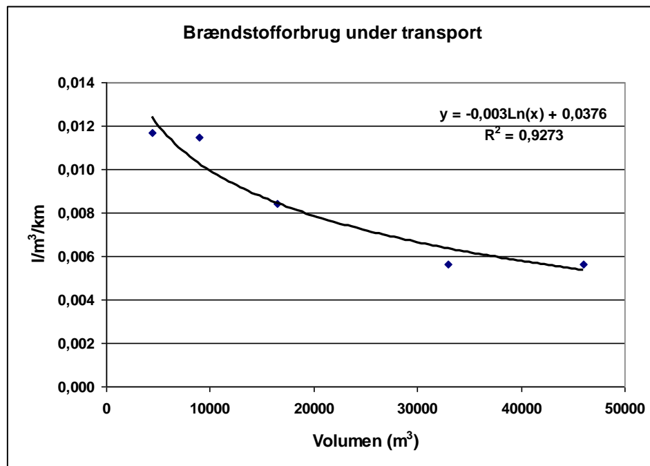
Figur 3.3 Relation mellem lastevolumen og brændstofforbrug for slæbesugere under indvinding og fuldladet transport.
