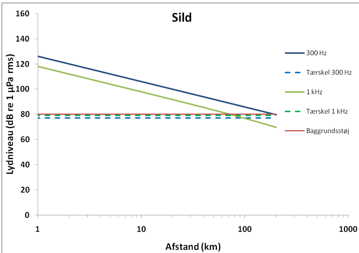
Figur 3: Silde detektionsafstand af en imaginær støjkilde (300 Hz og 1 kHz) og en kildestyrke på 190 dB re 1 μPa rms (1/3 oktav-bånd) 1m. Lydtrykkets aftagen som funktion af afstanden er afbilledet for frekvenser detekterbare for sild. Høretærsklerne for sild (Nedwell et al, 2004) er indtegnet som vandrette streger. Desuden er baggrundsstøjen indtegnet som en rød streg.
