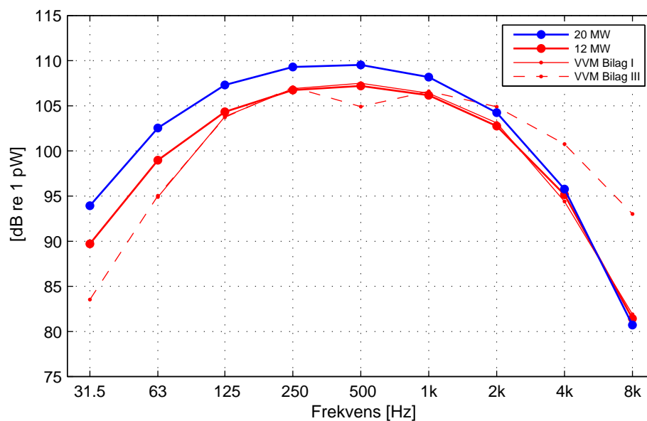
Figur 1. A-vægtede kildespektre for projektmøller på 12 MW (blå) og 20 MW (rød). Kildespektre benyttet i VVM-redegørelsens Bilag I og Bilag III er vist med tynd rød linje, henholdsvis fuldt optrukket og stiptet.
