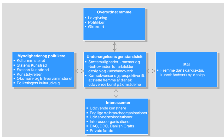
Figur 1.1: Undersøgelsens referenceramme
