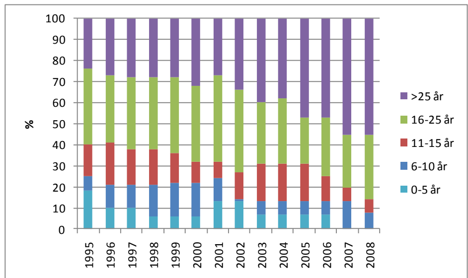
Figur 7. Aldersfordeling af de centrale kraftværker.
