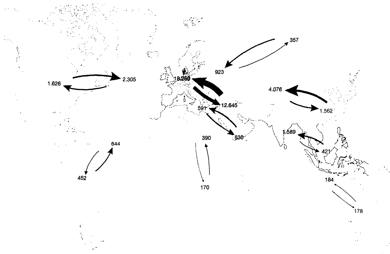
Figur 4: Handelsstrømmene målt i CO 2 -udledning 2001. Alle tal er i 1.000 tons. Pilene der peger væk fra Danmark viser den CO 2 -udledning Danmark har udledt for at producere eksportvarer til resten af verden. Pilene der peger hen imod Danmark viser den CO 2 -udledning der er sket i de forskellige verdensdele for at producere importvarer til Danmark.
