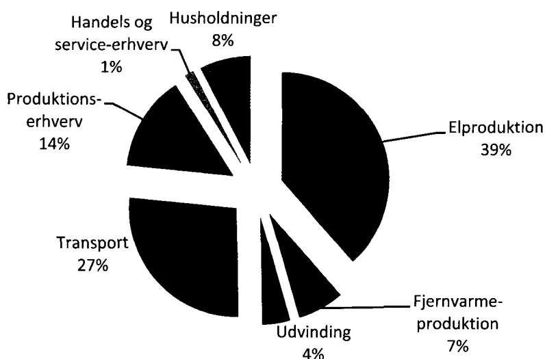
Figur 1: Danmarks CO 2 -udledninger 2001, Energistyrelsen 2002:30 (faktiske emissioner).
