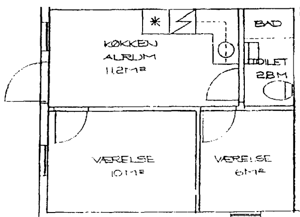
Plantegning af 30 m 2 lejlighed på Brovst Asylcenter. 24 lejligheder har værelser på 10 m 2 og 6 m 2 som vist. 12 andre lejligheder har to værelser på hver 8 m 2 .
