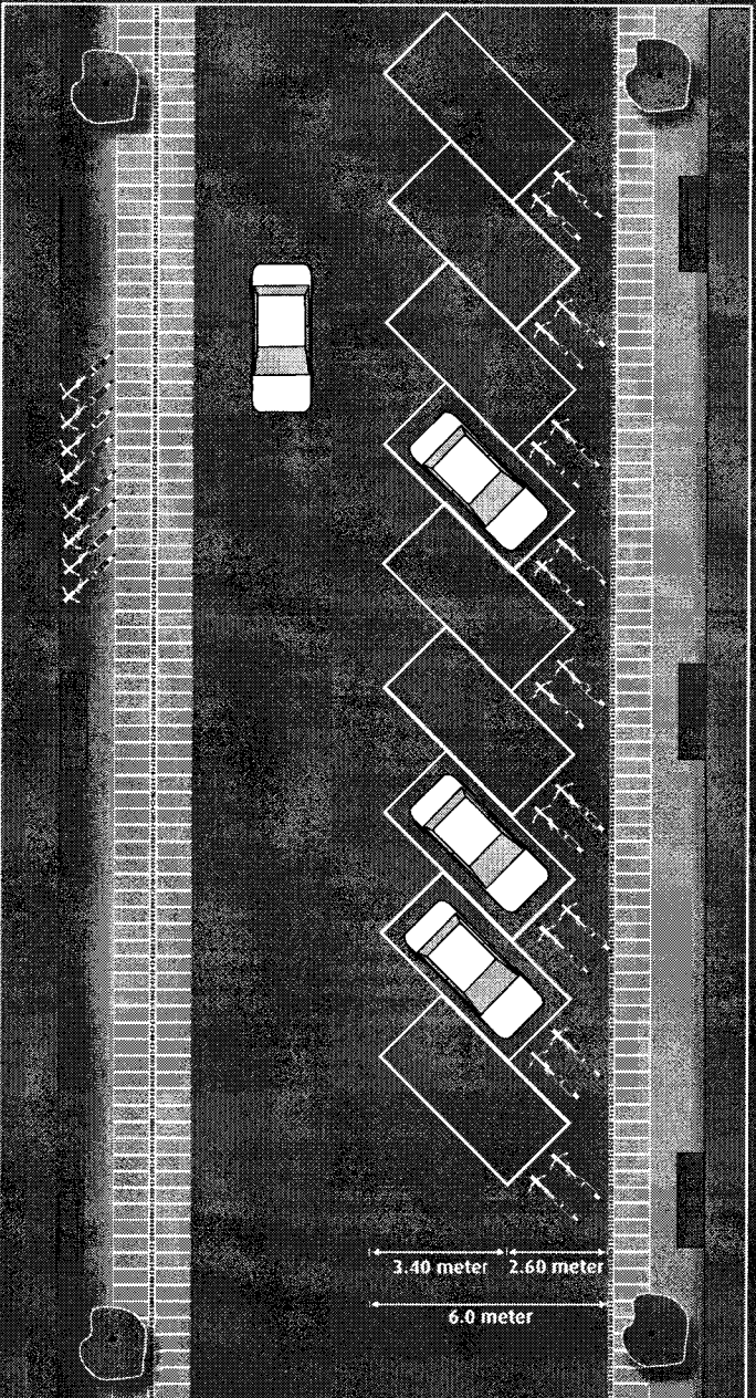
Udnyttelse af restarealer ved 45 graders skråparkering
