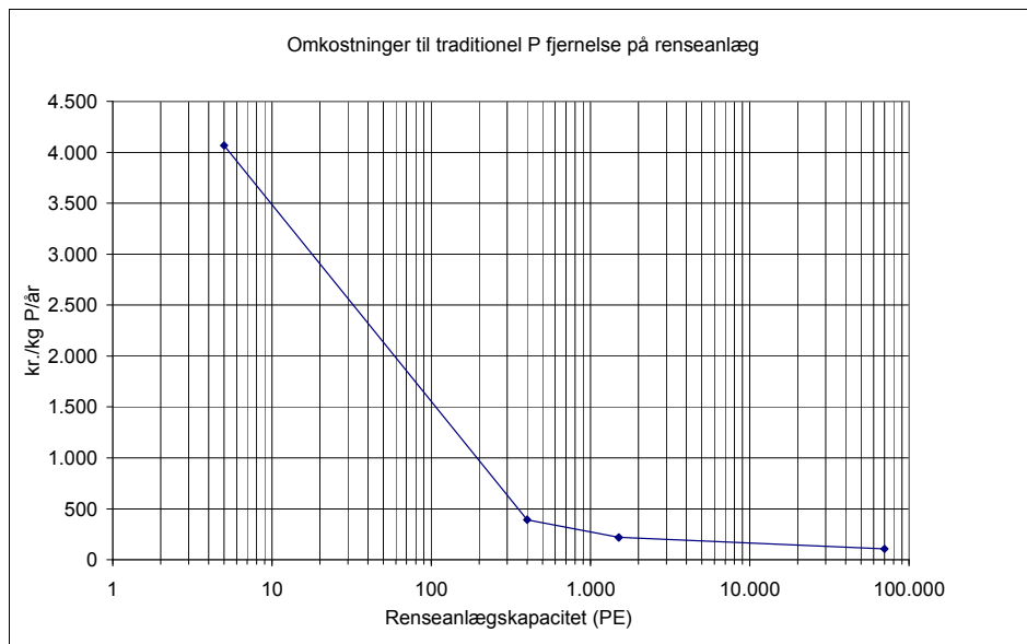
Figur 2.4 Sammenhæng mellem omkostninger til fjernelse af fosfor og renselæggenes størrelse/kapacitet almindelig kemisk fældning til ca. 0,5 mg/l).
