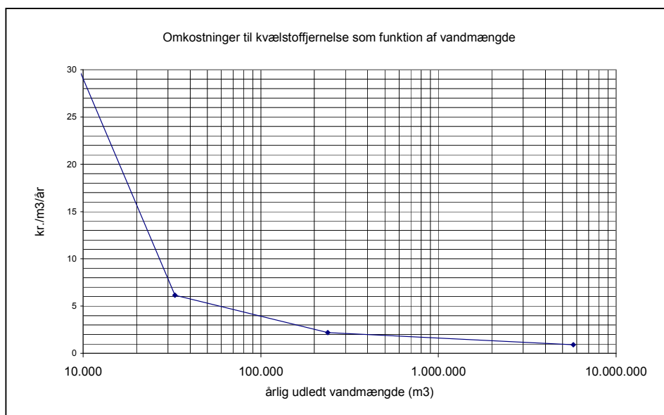
Figur 3.4 Sammenhæng mellem vandmængde tilført rensanlæg og omkostninger til kvælstoffjernelse regnet pr. m 3 /år.
