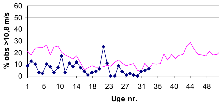
Figur 4 Hyppigheden af observationer pr. uge i 2006 af vindstyrker over 10,8 m/s svarende til hård vind eller mere (forbundne punkter) sammenlignet med middel for perioden 1994-2005 (tynd kurve). Baseret på ugeberetninger fra DMI.
