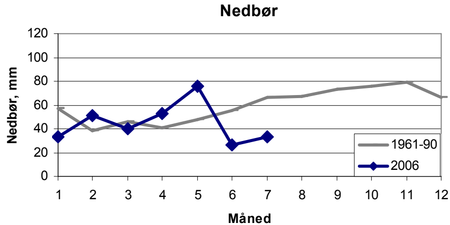
Figur 5 Månedlig nedbør i Danmark i 2006 sammenlignet med månedsmidler for perioden 1961-90. Baseret på månedsberetninger fra DMI.
