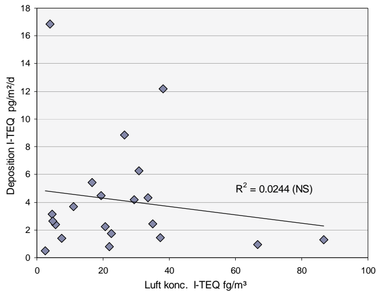
Figur 15. Der er ingen statistisk signifikant korrelation mellem PCDD/F i luft og deposition i Frederiksberg.
