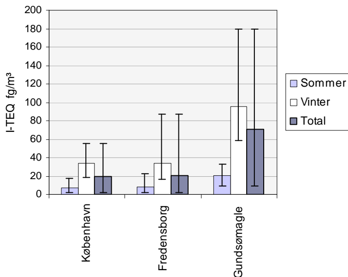
Figur 13. Deskriptiv statistik for PCDD/F i luft for alle stationer, hhv. sommer-, vinter- og samlet periode. Gennemsnit (vægtede med varighed), minimum og maksimum.
