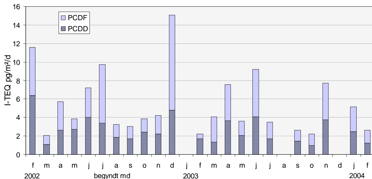
Figur 2. PCDD/F i gennemdrøp gennem grantræer ved Fredensborg 2002-2004
