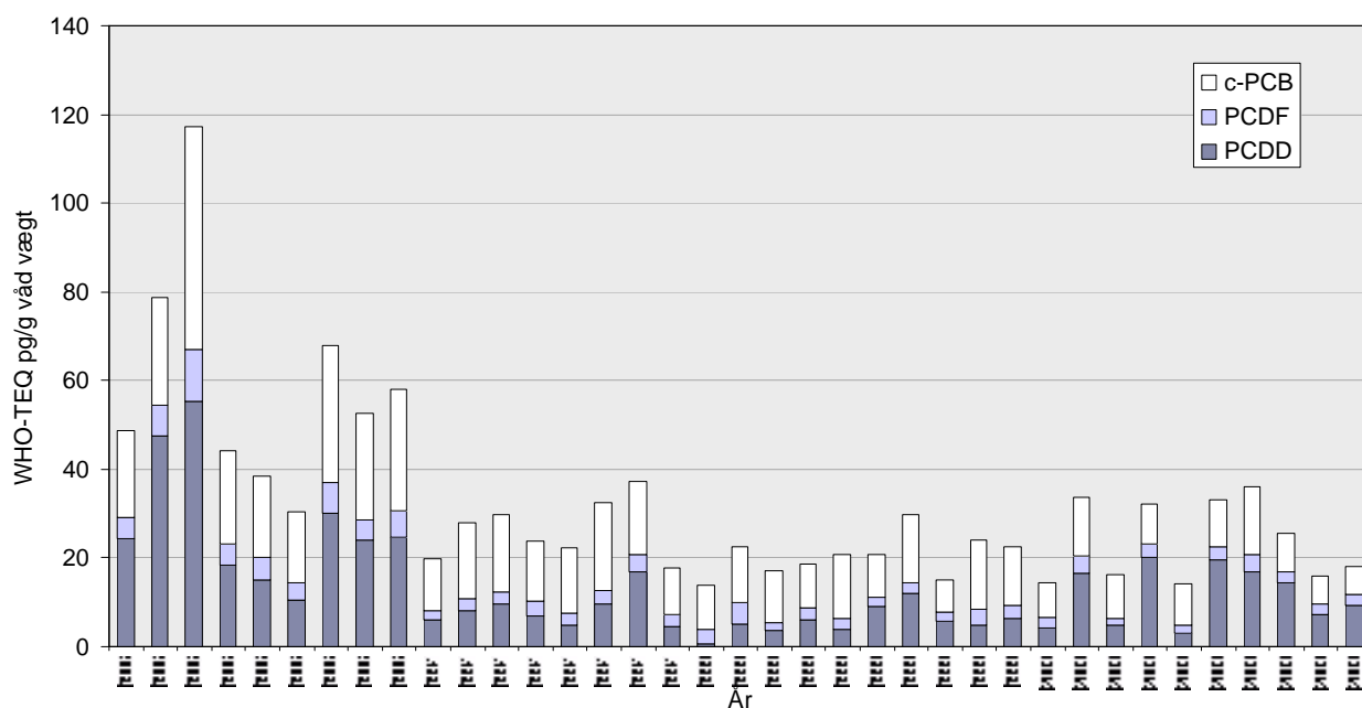
Figur 19 PCDD, PCDF og c-PCB i sælspæk fra Ittoqqortoormiit 1986-2003.
