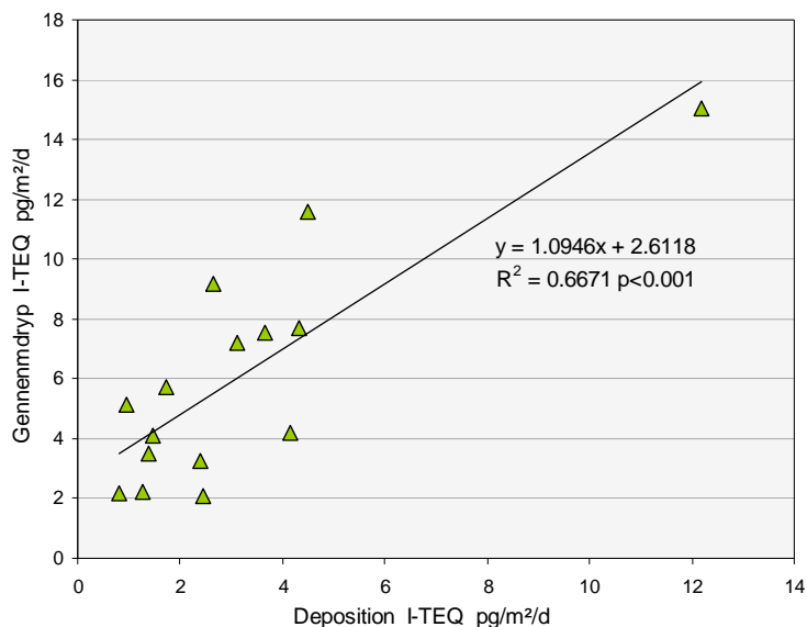
Figur 3. Der er en statistisk høj signifikant korrelation mellem PCDD/F i deposition og gennemdrøp i Fredensborg. Hældningen nær 1 viser at der er en nær sammenhæng mellem deposition og gennemdrøp, og at værdierne i store træk ligger på samme niveau med gennemdrøp 2,6 pg/m 2 /d højere.
