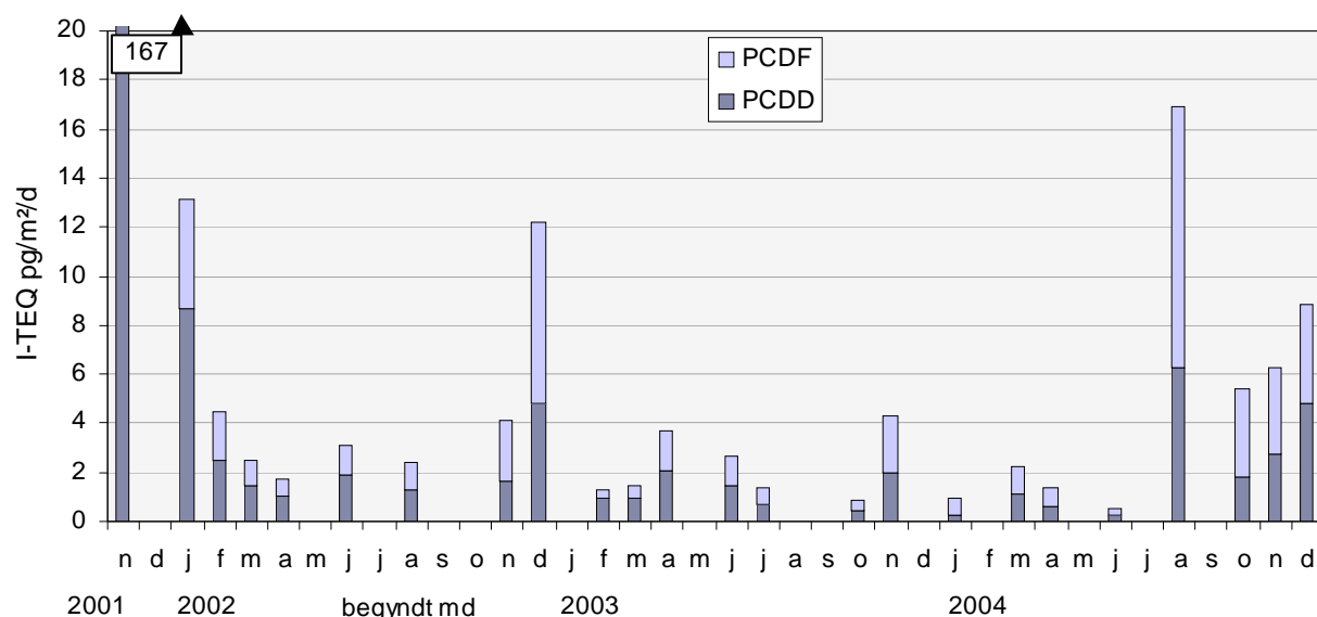
Figur 1. PCDD/F i deposition ved Roskilde nov.2001-jan. 2002, Fredensborg 2002-03. Sommer prøver er sammenblandet (pooleet) af flere enkeltprøver, anført ved begyndelsesmåned.
